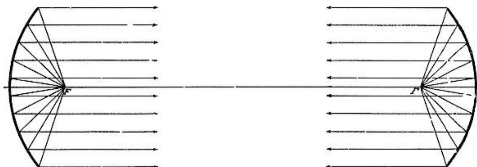
Parabolische Hohlspiegel-Anordnung nach Busse-Krall.
